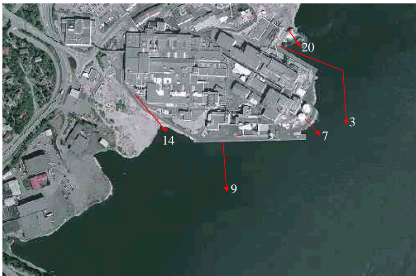
Figur 4. De fem utslippspunktene for prosessvann fra Glencore Nikkelverk AS er markert som punkt 3, 7, 9, 14 og 20 (fra Næs og Håvardstun 2013). Avløpsvann fra utslippspunktene 14 og 20 slippes ut på ca. 1 m dyp, mens avløpsvann fra utslippspunktene 3, 7 og 9 slippes ut på ca. 21 til 23 m dyp.
